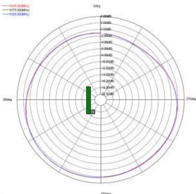
XY-PLANE
